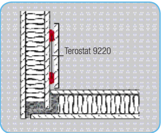
Merevítő elemek ragasztása konténergéjtátsnál és az autóiipari karosszéria géjtátsnál
